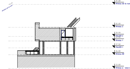
Elevation Sud m 1 : 100
