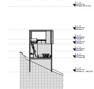
Coupe 1 m 1 : 100
