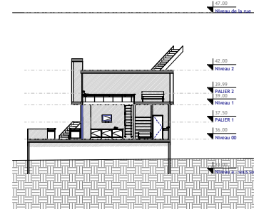
Coupe 0 m 1 : 100
