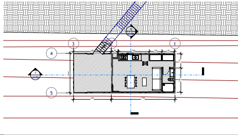
Niveau 00 m 1 : 100
